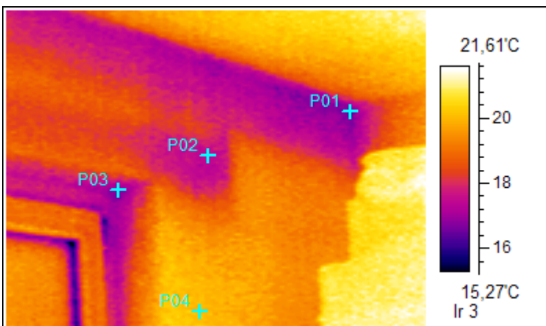
3. Zimmer 1 OG, Wandixel mit Abzeichnung des Ringbalkens und des Fenstersturzes
