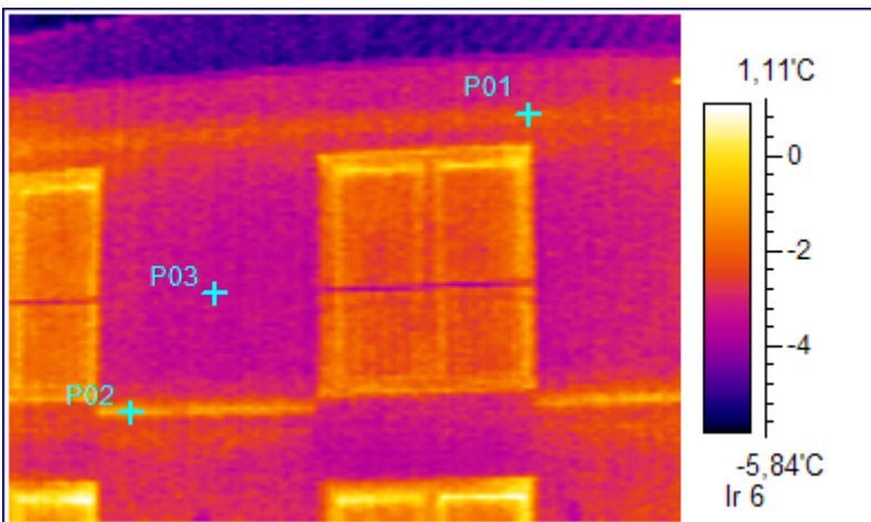
6. Fassade OG, Südseite mit Abzeichnung der Decke über EG und Ringbalken über OG
