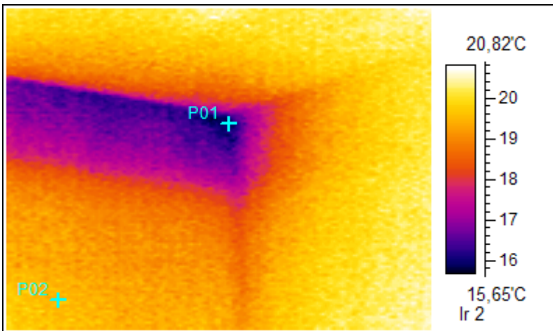
2. Schlafzimmer OG, Wandixel, Abzeichnung des Ringbalkens
