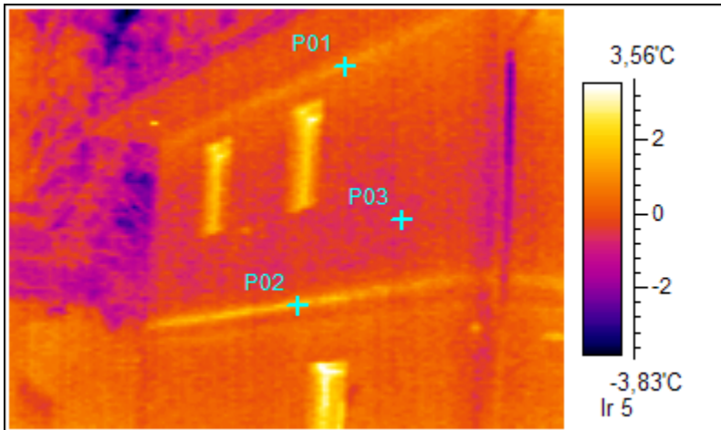
5. Fassade Ostseite, Südseite mit Abzeichnung der Decke über EG und Ringbalken über OG
