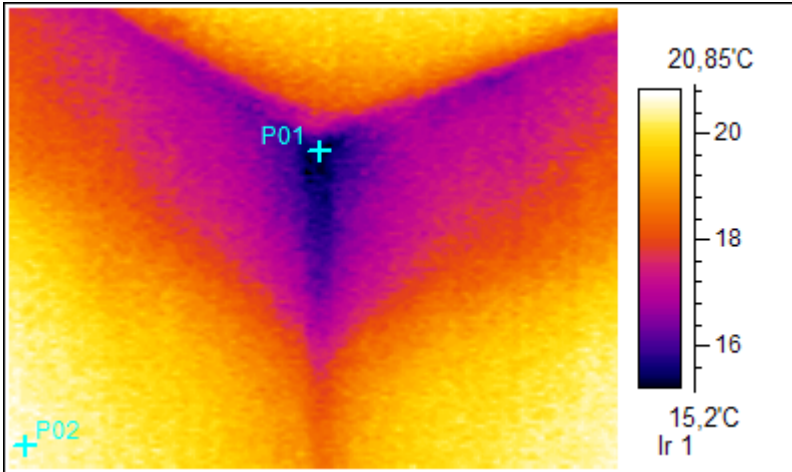
1. Schlafzimmer OG, Wandixel an der Außenwanddecke
