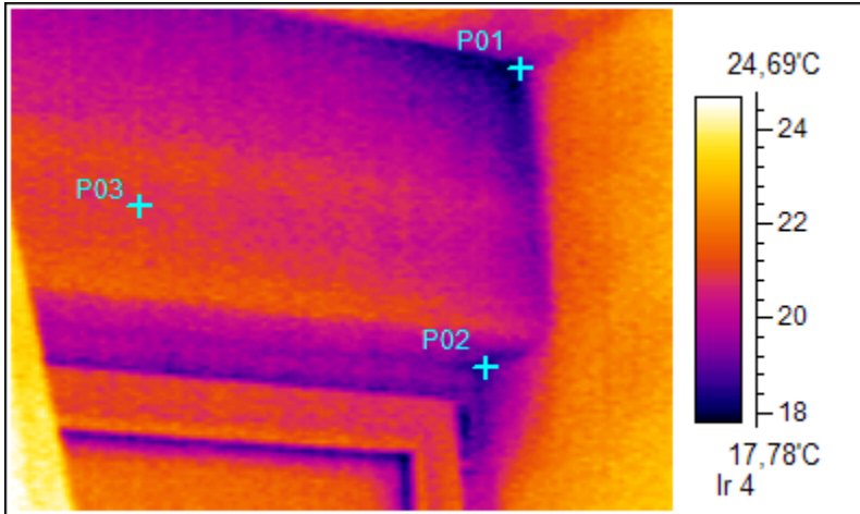
4. Bad OG, Fenstersturz rechts
